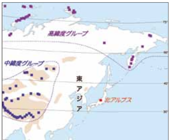
ユーラシア東部の氷河分布 (Polar Remote Sensing/GI/UAF, Zemp et al.(2014) から編図)
