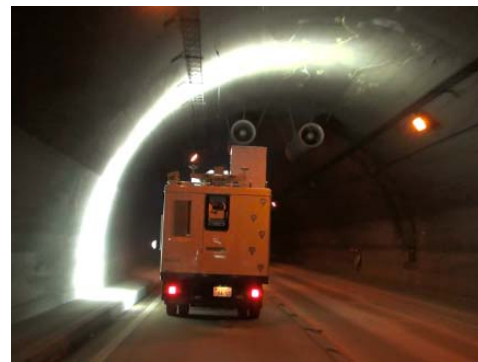
走行型高速 3D トンネル点検システム
