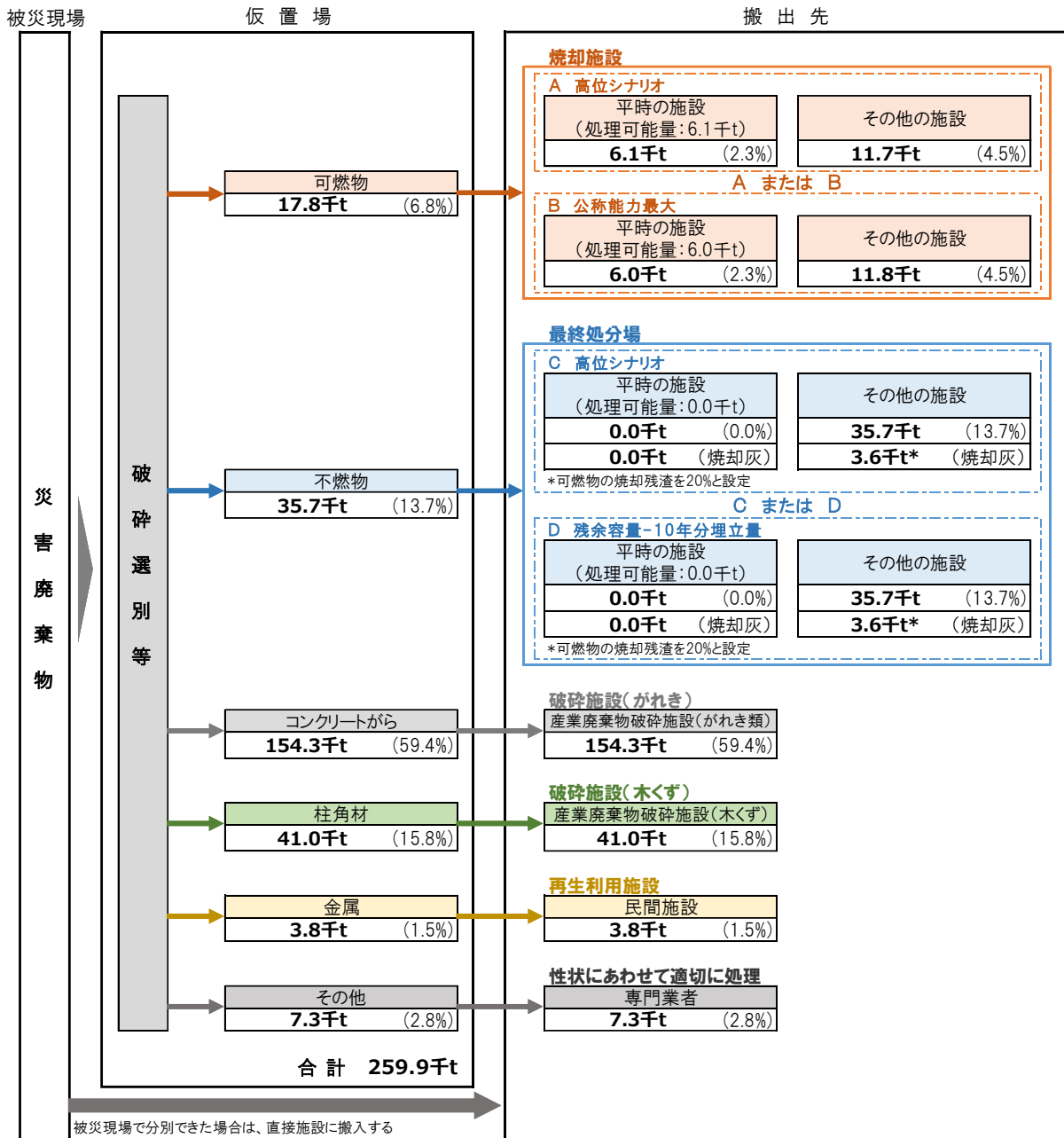
図2-6-8 糸魚川静岡構造線断層帯（全体）地震の災害廃棄物処理フロー（例）
