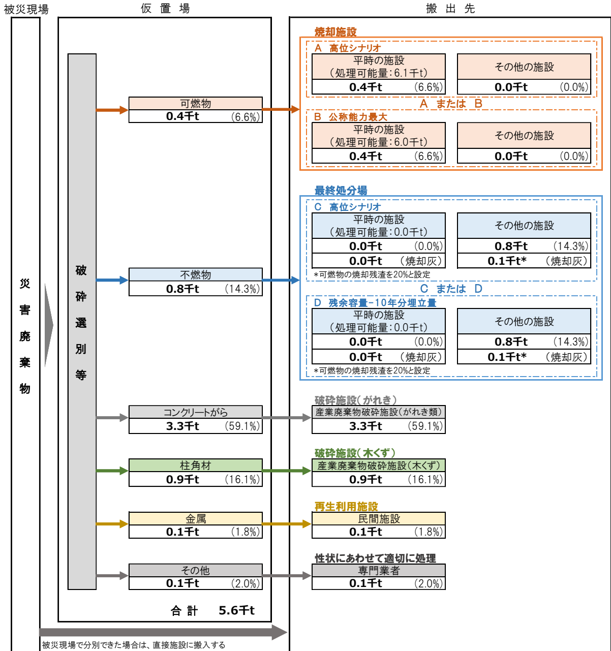
図 2-6-10 長野盆地西縁断層帯地震の災害廃棄物処理フロー (例)
