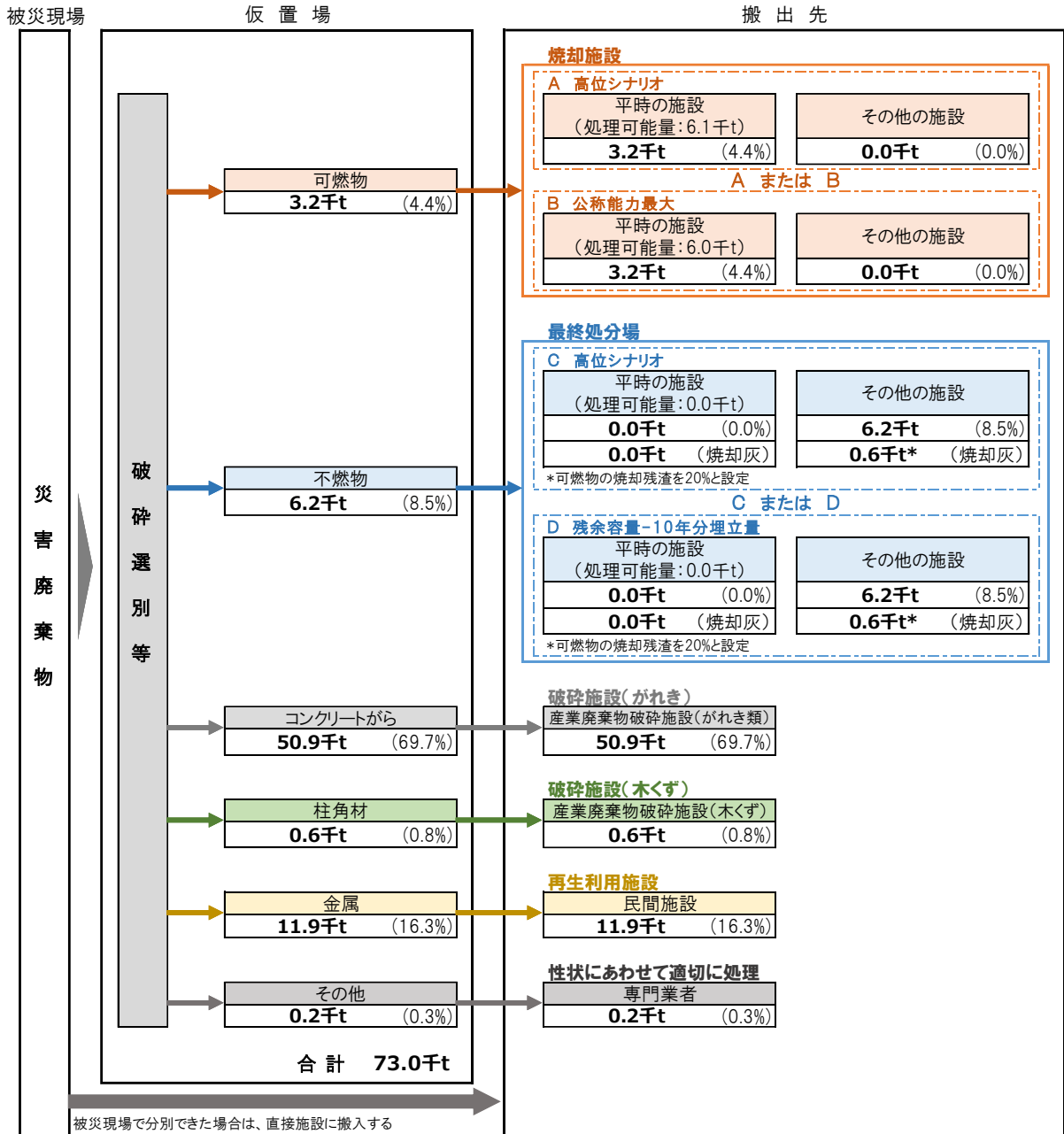
図 2-6-11 高瀬川・犀川計画規模降雨に伴う水害の災害廃棄物処理フロー (例)
