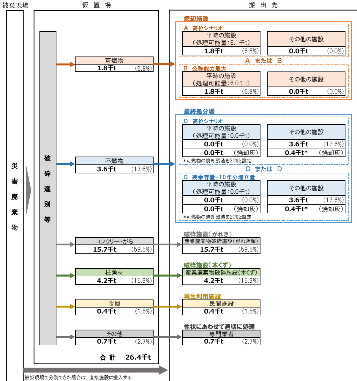
図 2-6-9 糸魚川静岡構造線断層帯（北側）地震の災害廃棄物処理フロー（例）
