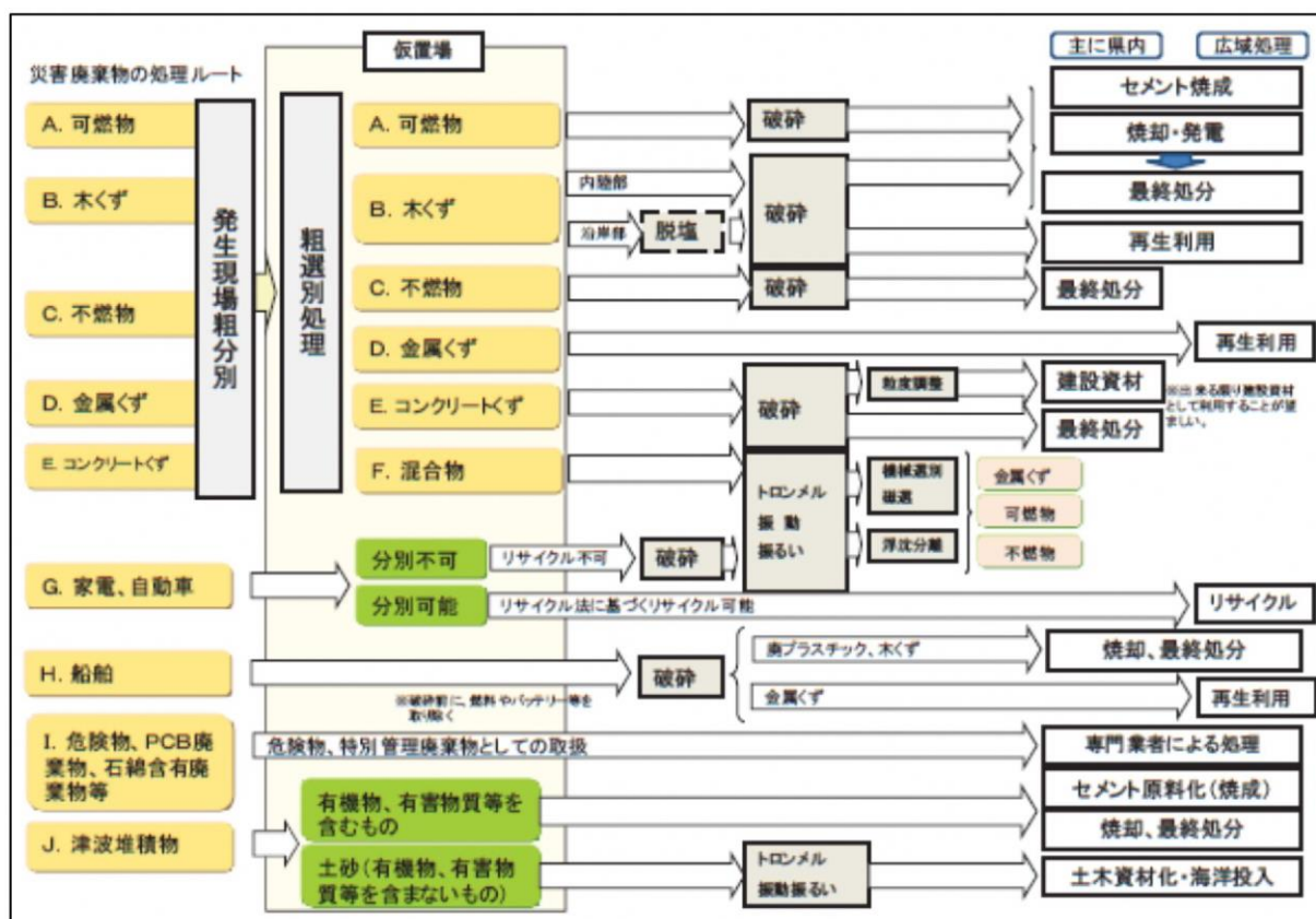
図 2-6-12 標準的な処理フロー
