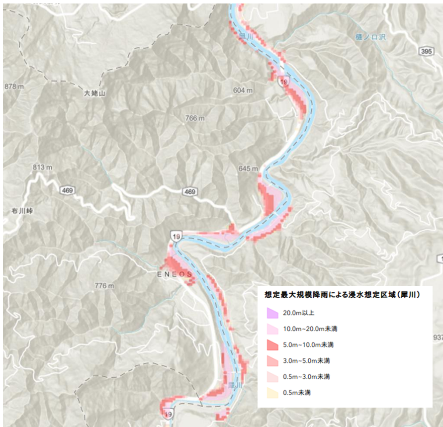
図 1-3-2 設定した浸水想定区域（犀川流域）
